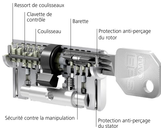
Cylindre à profil européen
