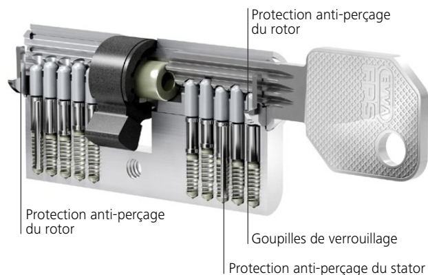
Cylindre à profil européen
